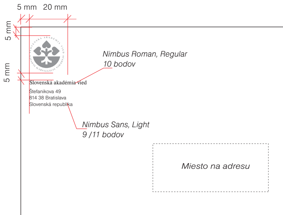
Poštová obálka štandardná, formát A6
